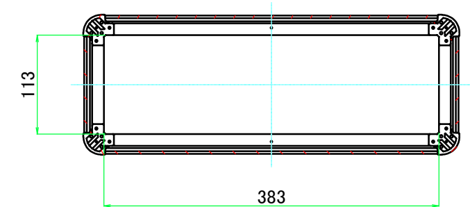
C-C ( 1 : 6 )
